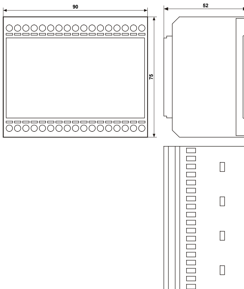
Rozmerový náčrt modulu POSIG3
